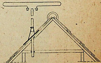
Montageplaat voor bevestiging van TV en FM antennes op schuine kappen
